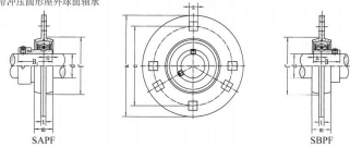
带冲压圆弧形外球面轴承
